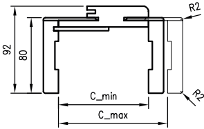
Doorsnede ORB 075
