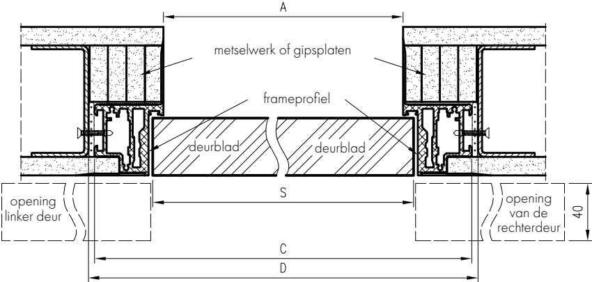
Doorsnede van Sara Eco2 flush - opening naar buiten
