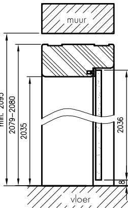
VERTICALE SECTIE OP VOOR GLAZEN DEUREN
