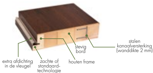
HERSE SECTIE 32 DB
