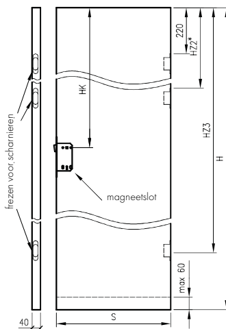
Deurblad vrij: Standard 10, Modern, Plus
