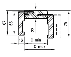
TUN sectie met hoek. T63
