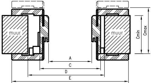
Horizontale doorsnedelste ORB
