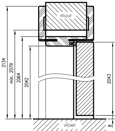
Verticale doorsnede van spanningsvrije deuren in ORB
