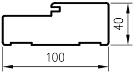
Profil OPB
