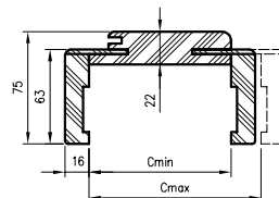
OR/ORC sectie met hoek. T63
