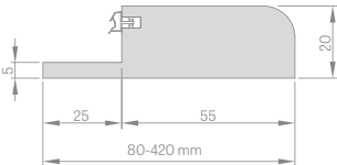
Hoek 6 cm en 8 cm
