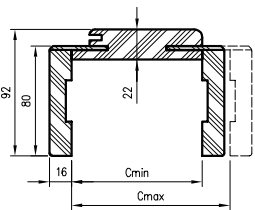
OR/ORC sectie met hoek. T80
