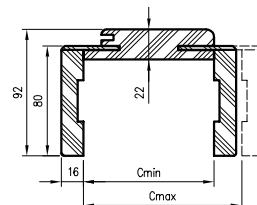
OR/ORC sectie met hoek. T80
