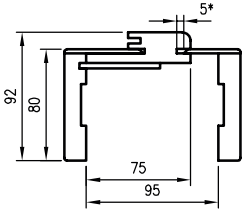
Doorsnede ORB 075
