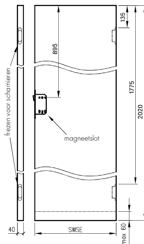
Sara Eco 2 deurbladen zonder korting in standaard 202X
