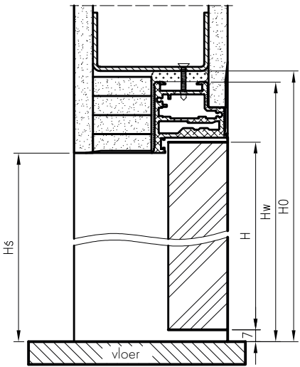
Verticale sectie Sara Eco 2 vlak - naar buiten openend
