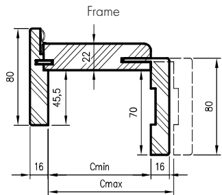
Horizontale doorsnede OF ORO
