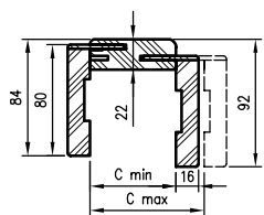
TUN sectie met hoek. T80
