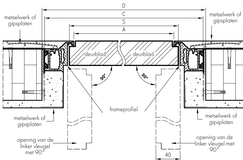
Doorsnede van Sara Eco2 sponningdeur - naar binnen openend
