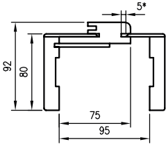
Doorsnede ORB 075
