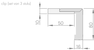
Hoek 6 cm en 8 cm
