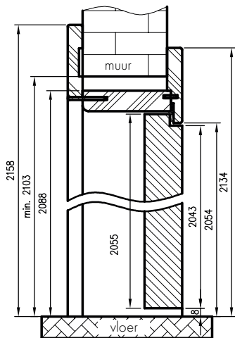
Verticale doorsnede ORO
