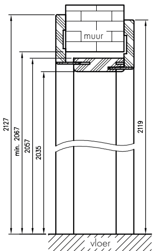
Verticale sectie van verstelbare tunnel met hoek. T80
