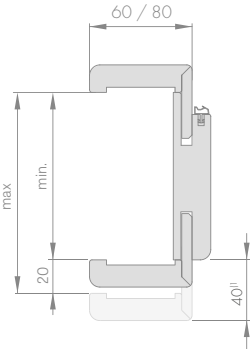
Verstelbereik van het verstelbare frame
