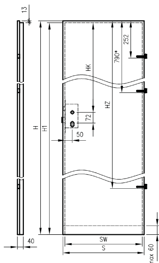
Deurblad vrij: Standard 10, Modern, Plus
