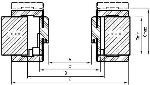
Horizontaal gedeelte ORB
