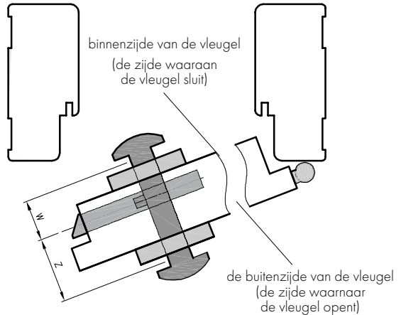
Selectie van de grootte van het inzetstuk met knop
