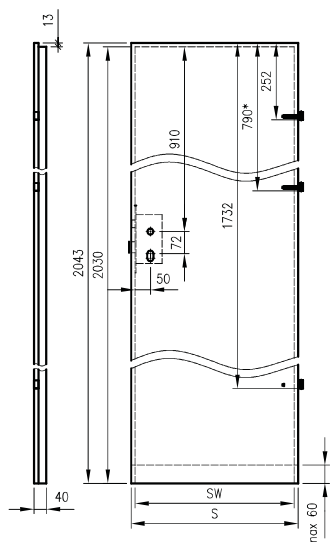
Draaivleugels zonder spanning
