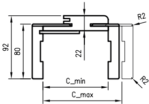
Doorsnede ORB 095-300
