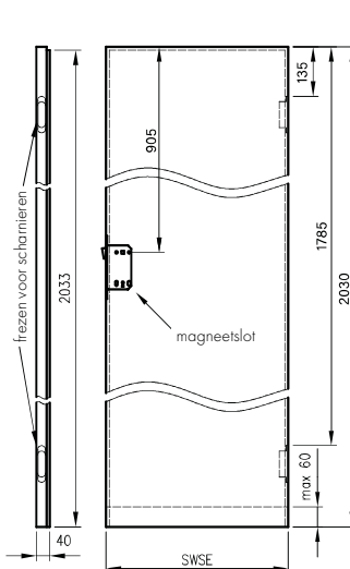
Beglaasde vleugels Sara Eco 2 Standaard 202X
