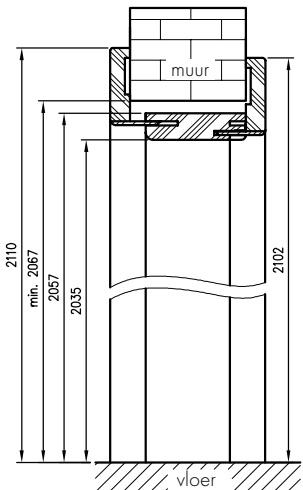
Verticale sectie van verstelbare tunnel met hoek. T63
