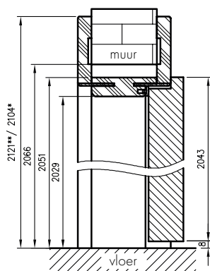
Verticale doorsnede van spinningdeur met OR
