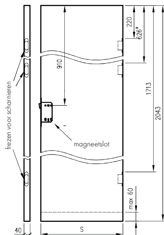
Draaivleugels zonder spanning
