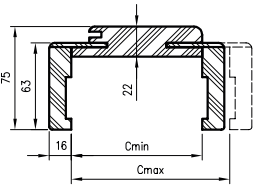
OR/ORC sectie met hoek. T63
