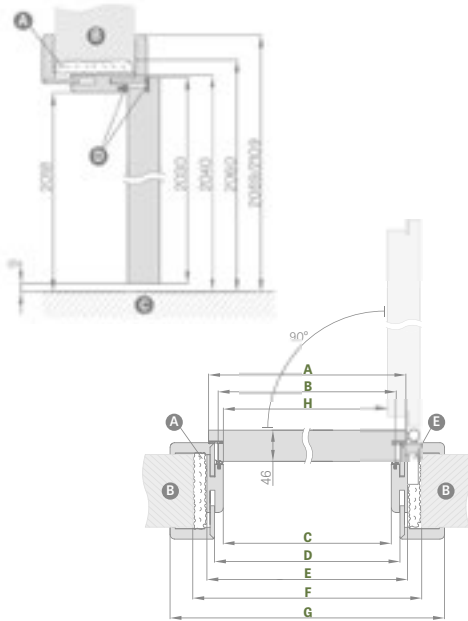
Verstelbaar frame diagram
