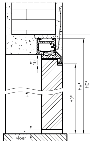
Doorsnede van Sara Eco2 sponningdeur - naar binnen openend
