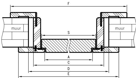
Horizontale doorsnede OF ORO
