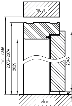
VERTICALE DOORSNEDE OP VOOR SPONNINGDEUREN
