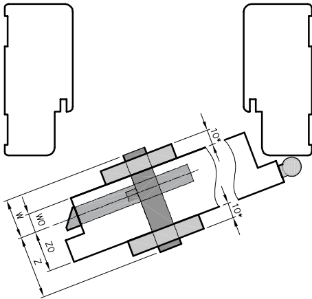
Dimensionering van de slotcilinder
