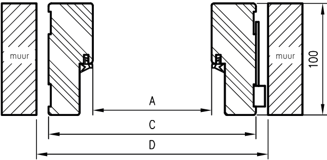
Horizontale doorsnede van de RDF
