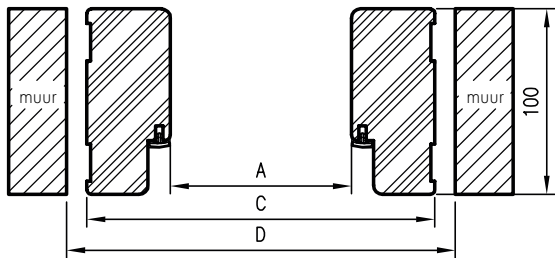
HORIZONTALE SECTIE OP
