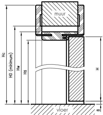
Verticale doorsnede ORB
